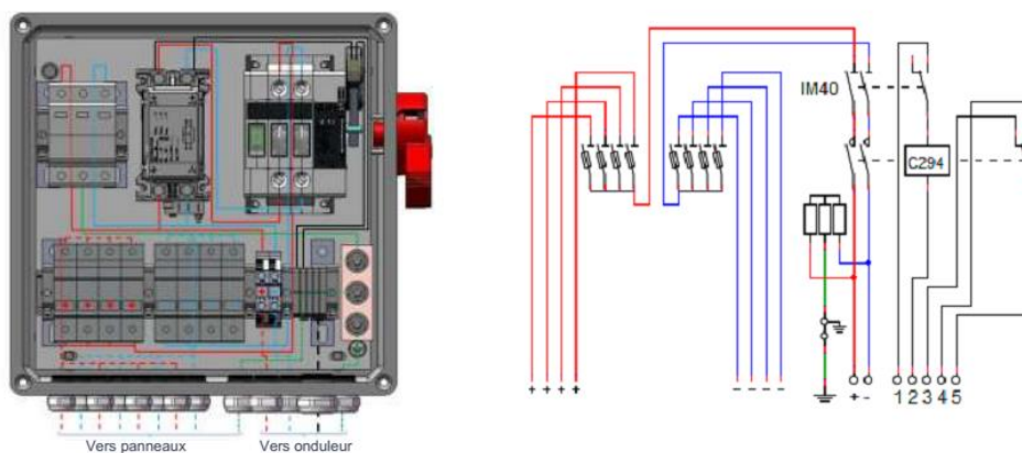
Boite de jonction PV 4 chaines 40A 1000V
